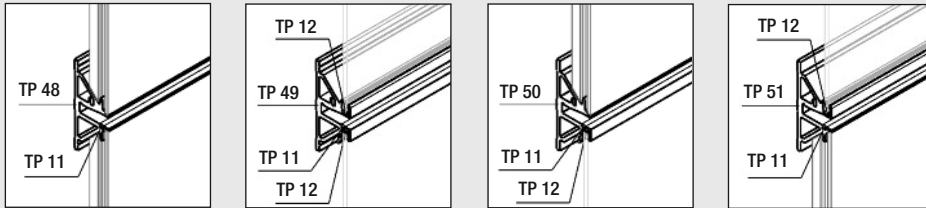
POSSIBILI SITUAZIONI DI INIZIO PANNELLATURA. SOLUTION OF STARTING PANEL.
