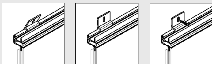
PARTICOLARE STAFFA DI FISSAGGIO (TP 13). DETAILS OF FIXING BRACKET (TP 13).
