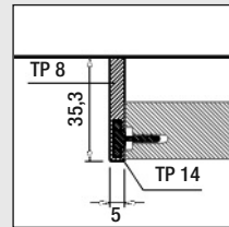
SEZIONE ORIZZONTALE. HORIZONTAL SECTION.
