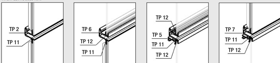
POSSIBILI SITUAZIONI INTERMEDIE. INTERMEDIATE SOLUTION.
