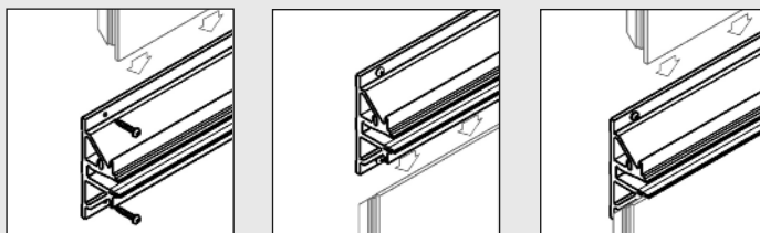
PARTICOLARE FISSAGGIO A PARETE CON PROFILI FORTI. DETAILS OF WALL FASTENING WITH STRONG PROFILES.
