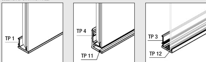
POSSIBILI SITUAZIONI DI INIZIO PANNELLATURA. SOLUTION OF STARTING PANEL.
